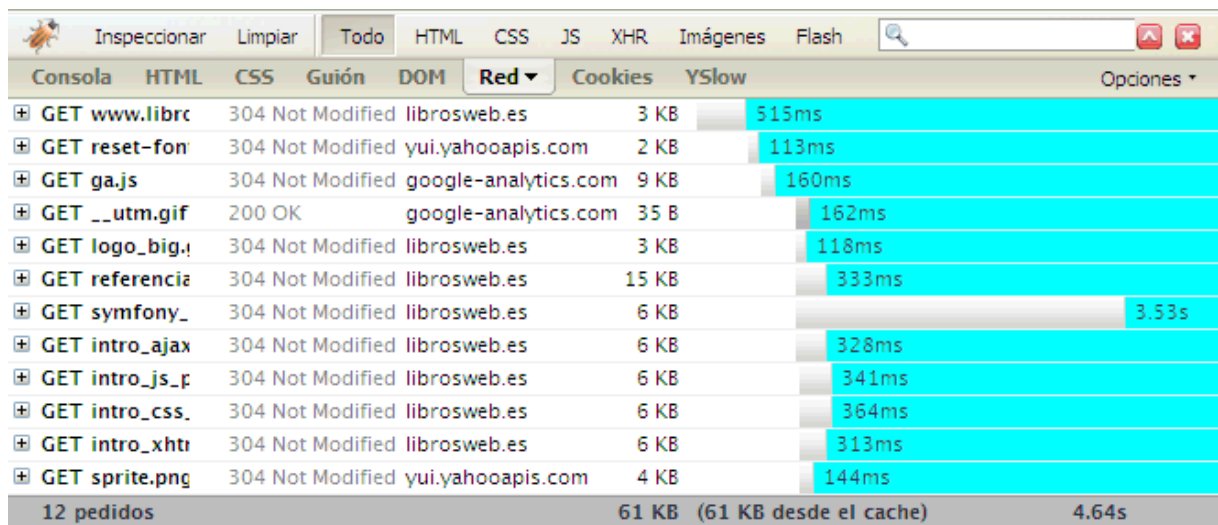
Figura 2.12. Panel Red de Firebug
